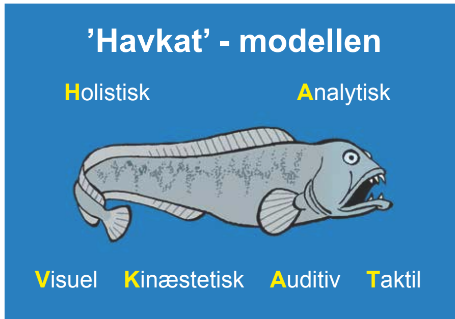
Figur 8: Havkat-modellen Havkat-modellen
